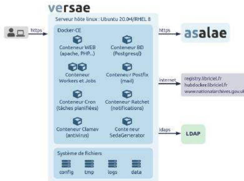
Schéma d'architecture technique Versae
