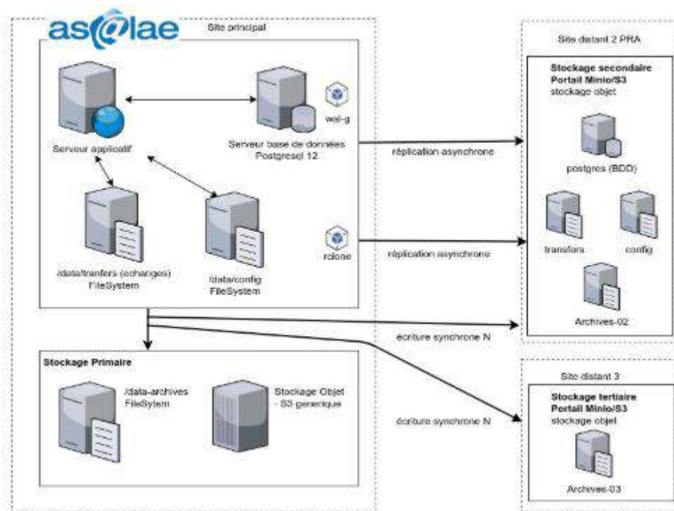
Schéma d'architecture réplication + écriture en N
