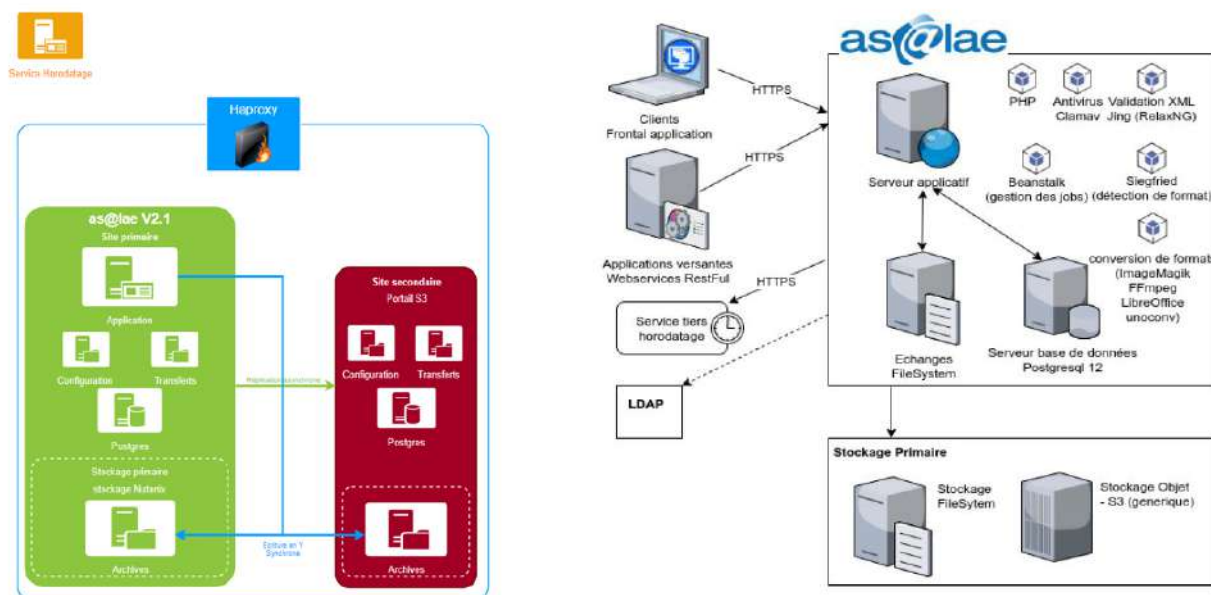
Schéma d'architecture technique Asalae
